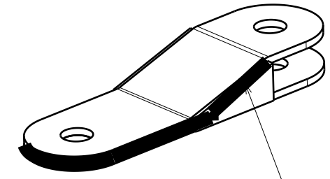
Cordon continu avec apport de matière
