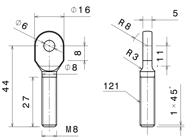
Vue de face Echelle : 1:1 Vue de gauche Echelle : 1:1
