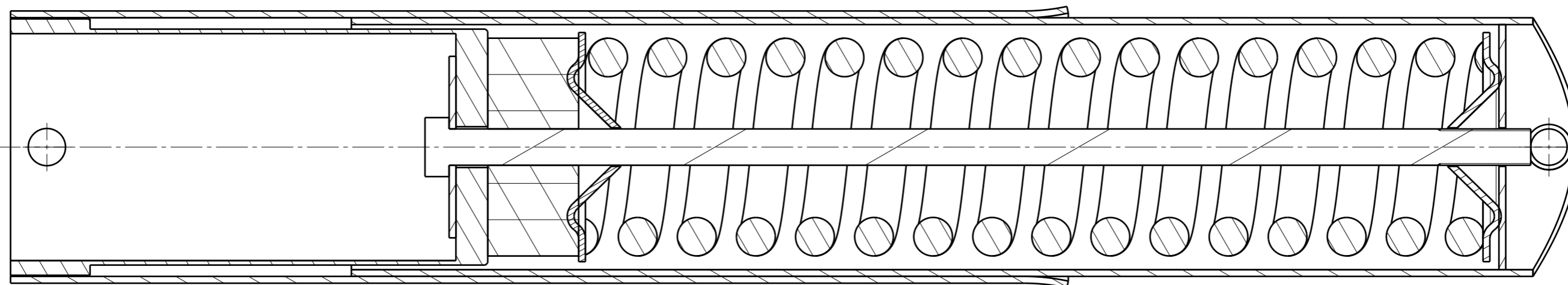
Coupe A-A Echelle : 1:1
